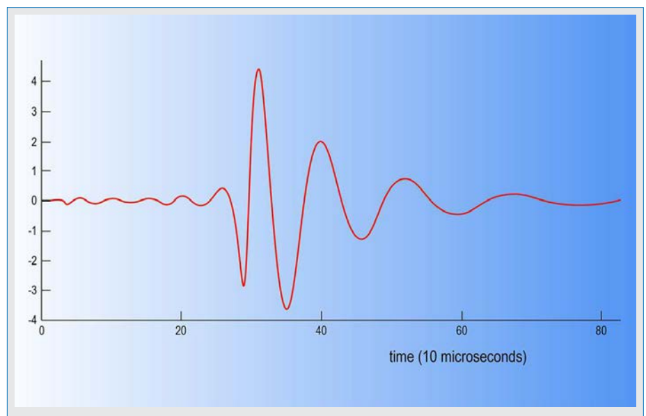
Abb. 2: Eine typische CD-Sferics-Frequenzform
