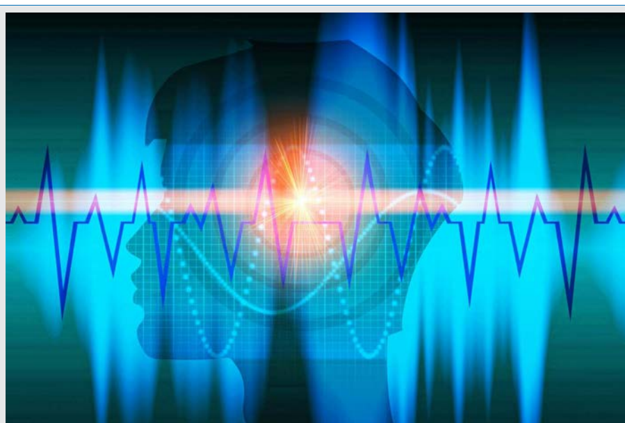
Abb. 1: Die Physik steuert die Biochemie
